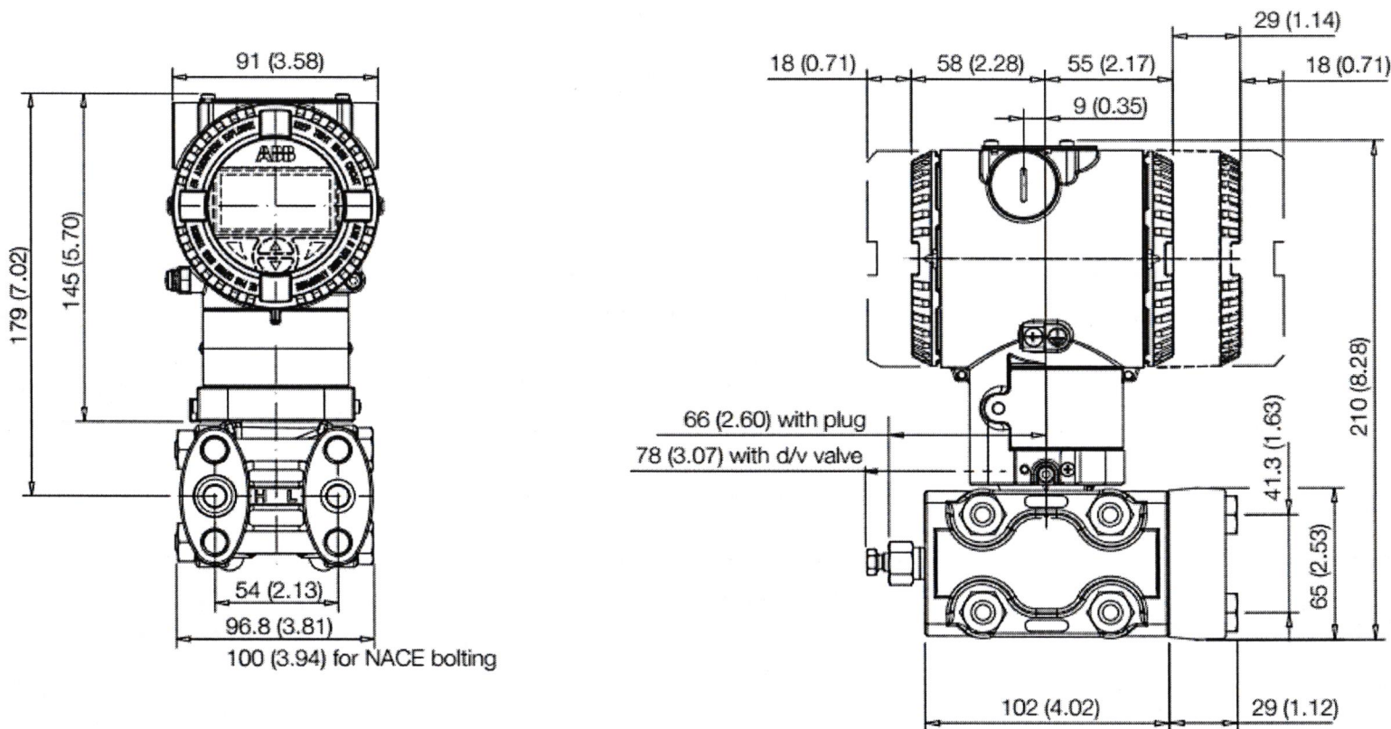
Размеры и распределение соединения/ Connection dimensions and distribution
